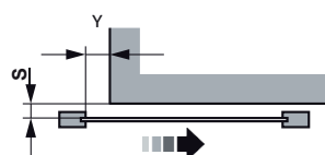
Protecció enfront de l'atrapament dels dits
